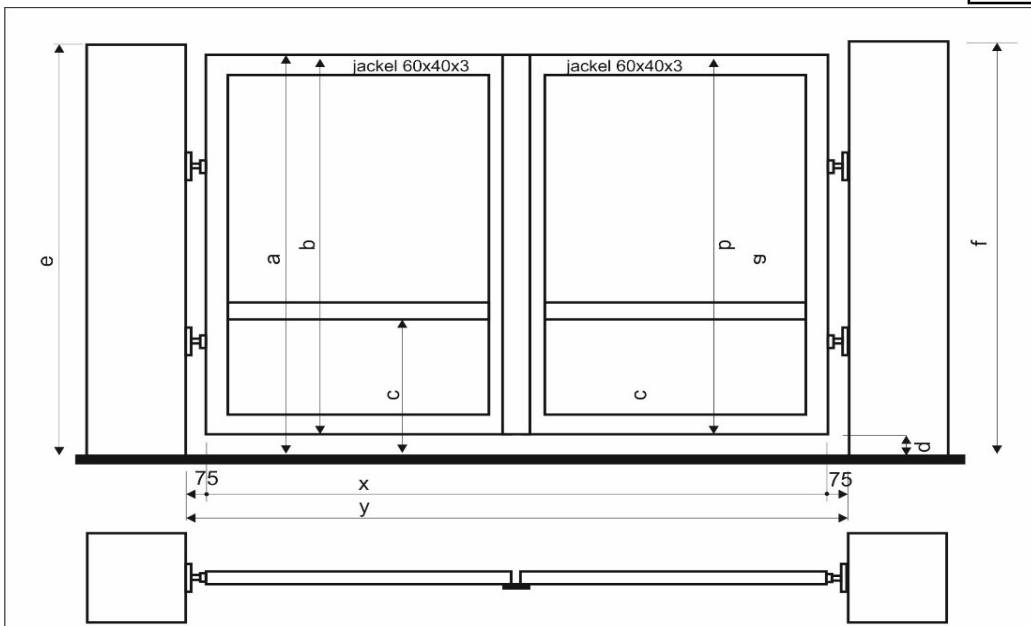
pohled na branku z ulice (otevírání dovnitř)
